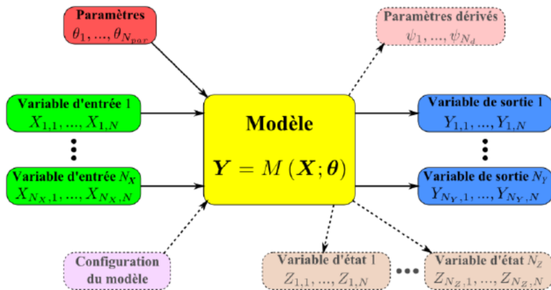
Schéma 1 : Bayesian Modeling
